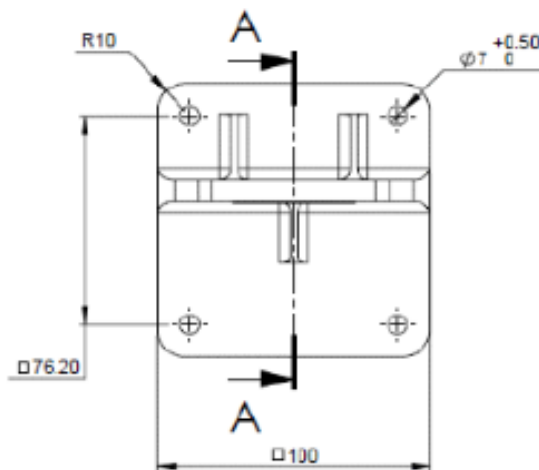
Рисунок 1: Основание наклонной крепежной базы - вид сзади
