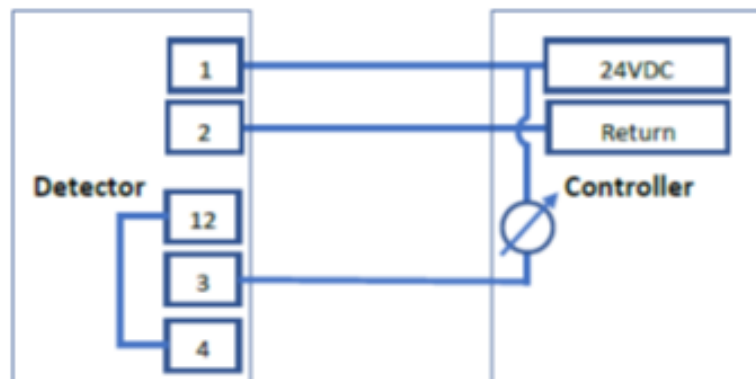
Рисунок 7 - 3-проводная схема поглотителя (Sink)
