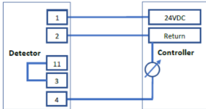
Рисунок 6: - 3-проводная схема источника (Source)
