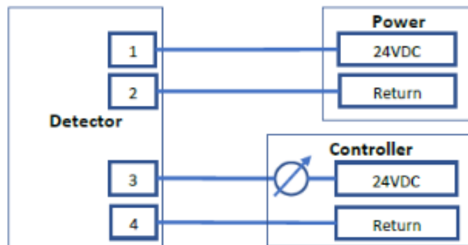
Рисунок 5: - 4-проводная схема поглотителя (Sink)
