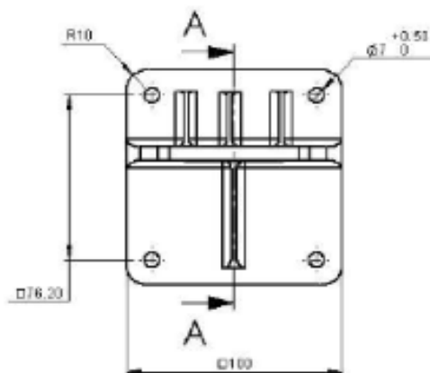
Рисунок 1: Основание наклонной крепежной базы - вид сзади
